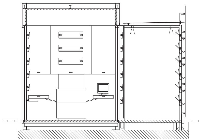
Sezione trasversale
