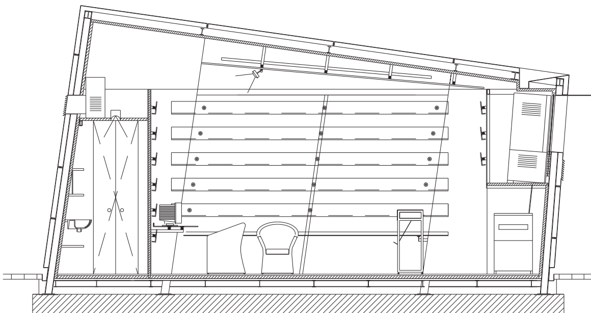
Sezione longitudinale
